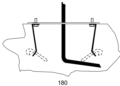
Montaż podstawy szlabanu
