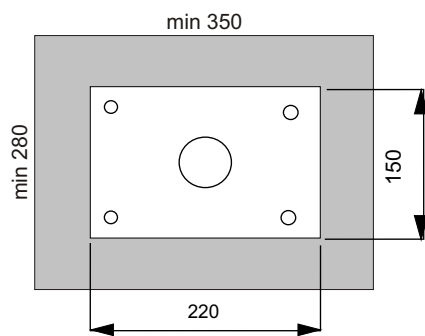
Wymiary fundamentu 350mm x 280mm
